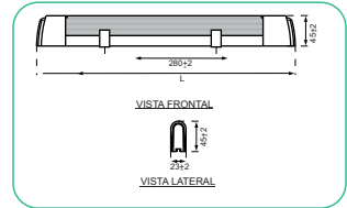
Dibujo (Dimensiones)
